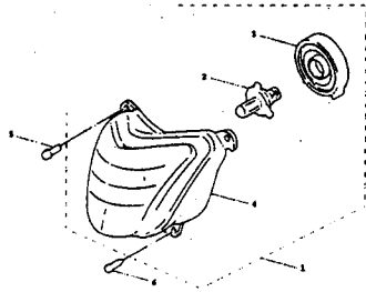
FIG. 40 前燈 ..... 140
