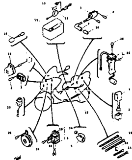
FIG. 43 電裝1 ..... 148
