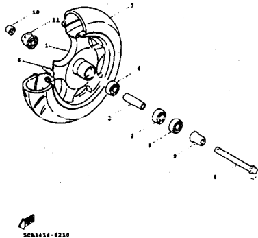
FIG. 25 前輪 ..... 90
