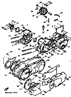
FIG. 13 傳動機構 ..... 50
