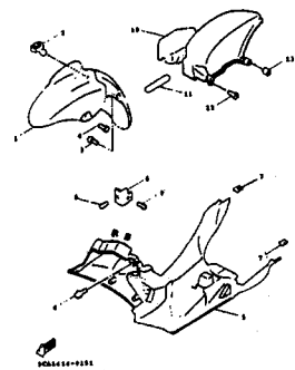
FIG. 18 側蓋 ..... 60
