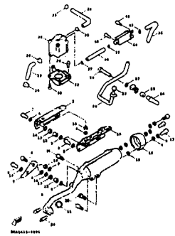
FIG. 9 排氣裝置 ..... 28
