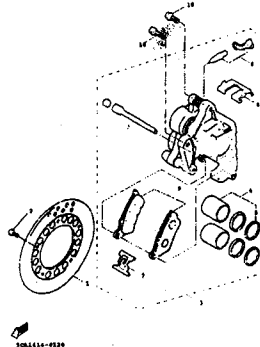
FIG. 26 前剎車卡鉗 ..... 92
