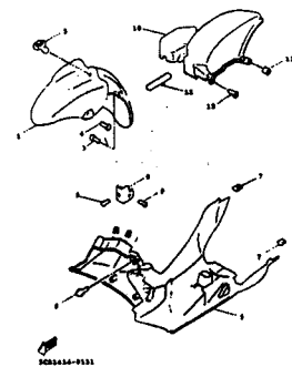
FIG. 17 擋泥蓋後架 ..... 58
