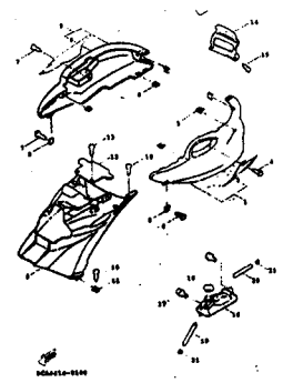
FIG. 18 側蓋 ..... 60
