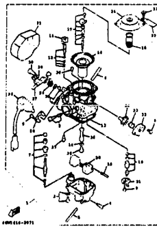
FIG. 8 化油器 ..... 24
