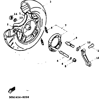
FIG. 27 後輪 ..... 94
