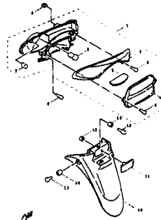
FIG. 41 後燈 ..... 142
